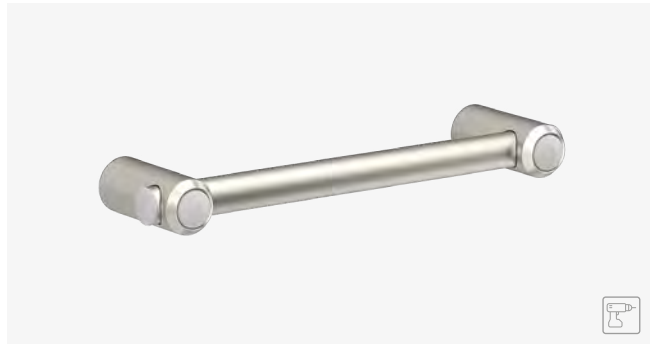
SHOWER GRAB BAR 400 MM. BARRA SEGURIDAD 400 MM SATIN STAINLESS STEEL A: 412 mm. B: 45 mm. C: 108 mm. D: 350 mm.
