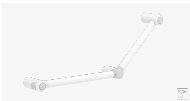
GRAB BAR ANGULAR 400X300 MM. BARRA SEGURIDAD ANGULAR 400X300 MM WHITE A: 436 mm. B: 336 mm. C: 108 mm.
