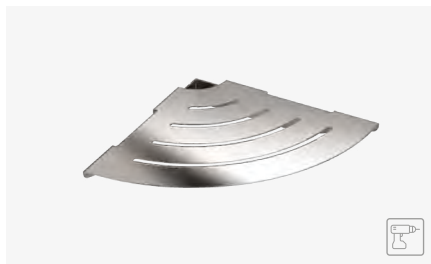
CORNER METAL SHELF REPISA METÁLICA ESQUINA SAT. ST. STEEL / INOX SATINADO POL. ST. STEEL / INOX PULIDO BLACK WHITE A: 220 mm. B:40 C: 220 mm. D: 90 mm.
